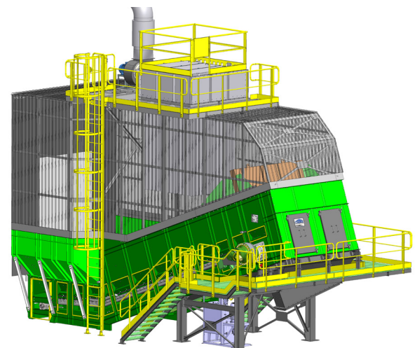
Descargador de camión diseñado con SOLIDWORKS
